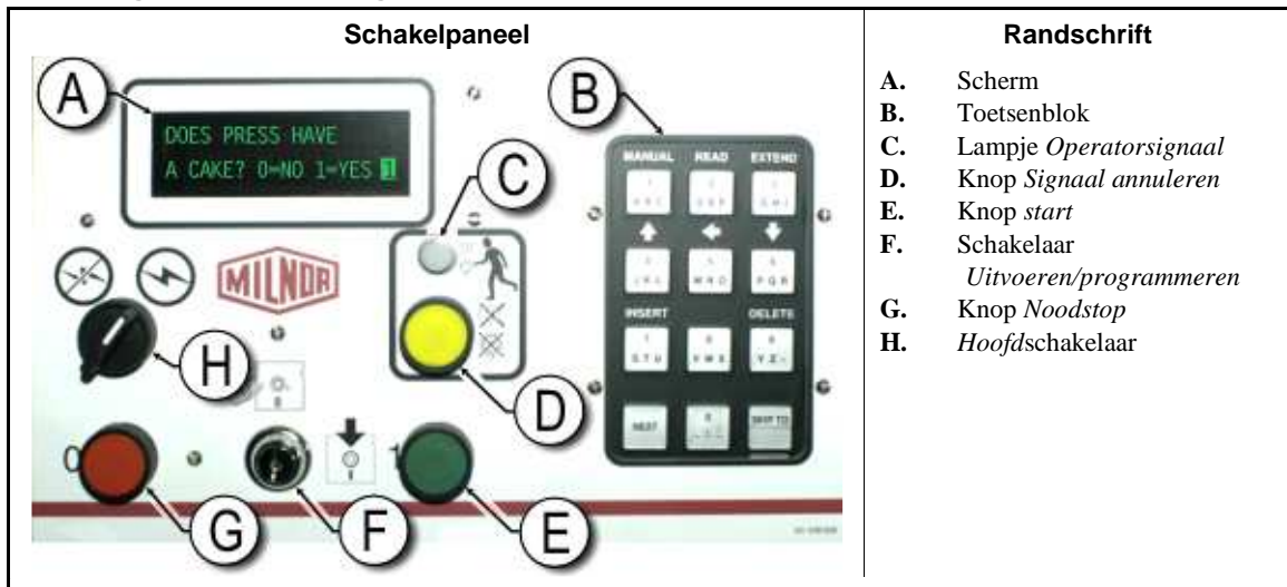
Afbeelding 2: Hoofdbedieningspaneel met toetsenblok met 12 knoppen
