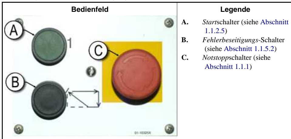
Abbildung 3: Stopp/Fehlerbeseitigung Steuerelemente
