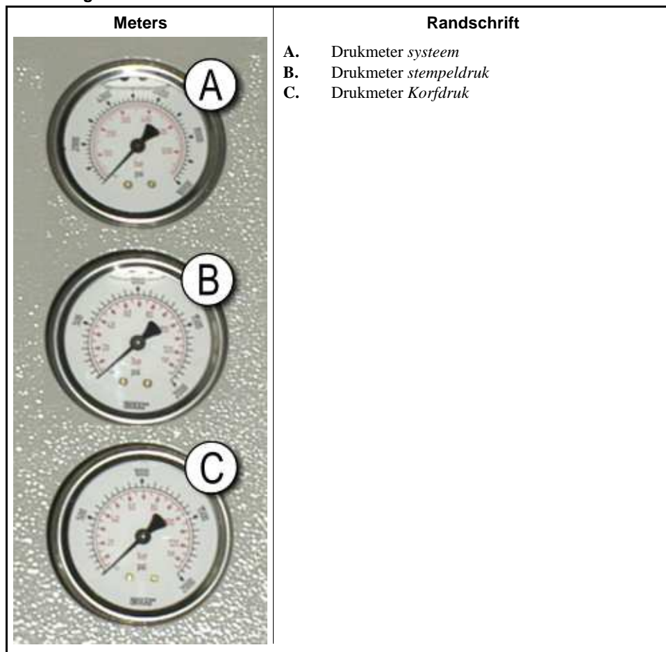
Afbeelding 7: Drukmeters
