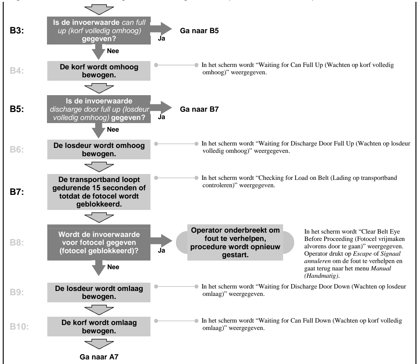
Programmakaart 1: Overzichtsdiaagram voor Evening Shutdown ('s Avonds uitschakelen)
