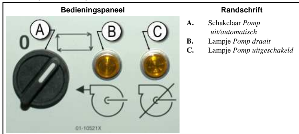
Afbeelding 4: Bedieningselementen Retourpomp
