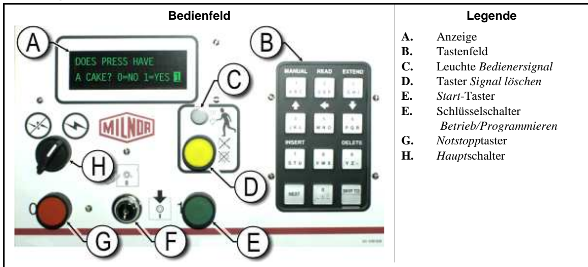
Abbildung 2: Hauptbedienfeld mit einer 12-Tasten-Tastenfeld
