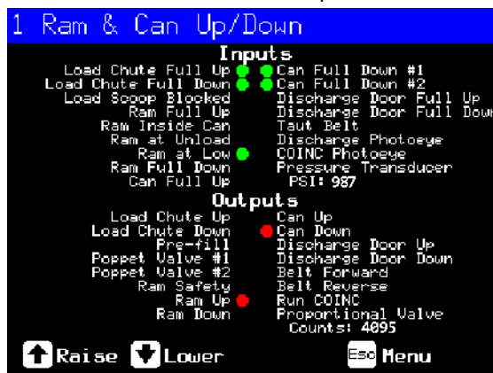
Illustration 16: Ecran 1 Vérin et panier en haut/bas
