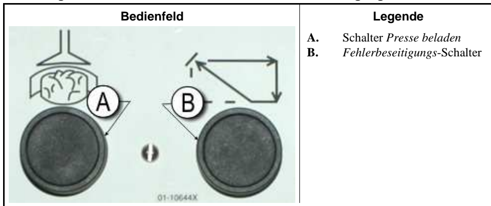
Abbildung 5: Steuerelemente „ Presse beladen/Fehlerbeseitigung “
