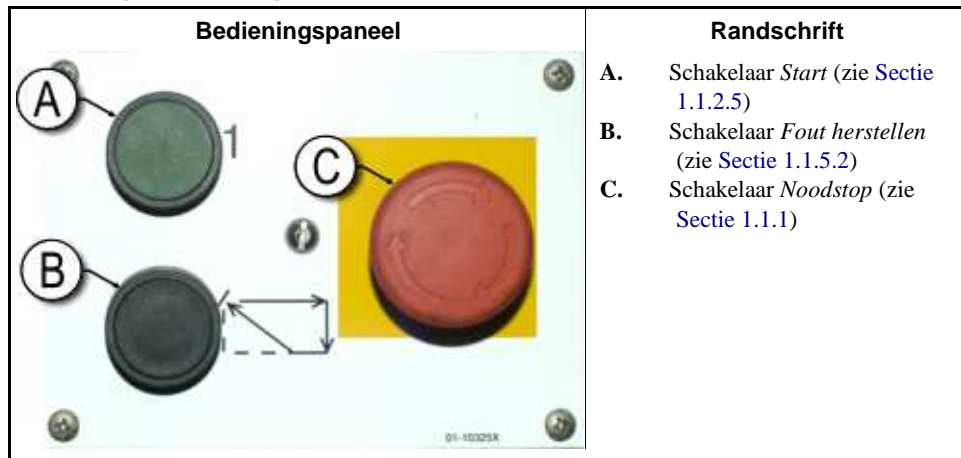
Afbeelding 3: Bedieningselementen Stop/Fout herstellen
