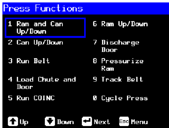
Illustration 15: Ecran de menu Fonctions de la presse
