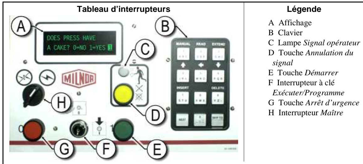
Illustration 2: Pupitre principal avec clavier 12 touches
