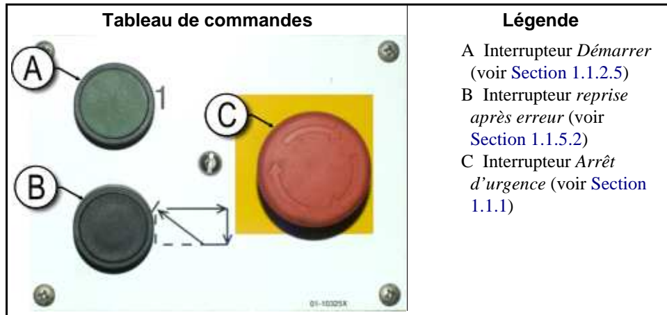
Illustration 3: Commandes Reprise après arrêt/erreur
