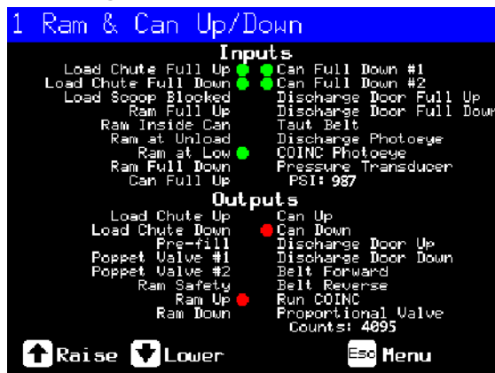
Afbeelding 16: Scherm 1 Ram and Can Up/Down (1 Stempel en korf omhoog/omlaag)
