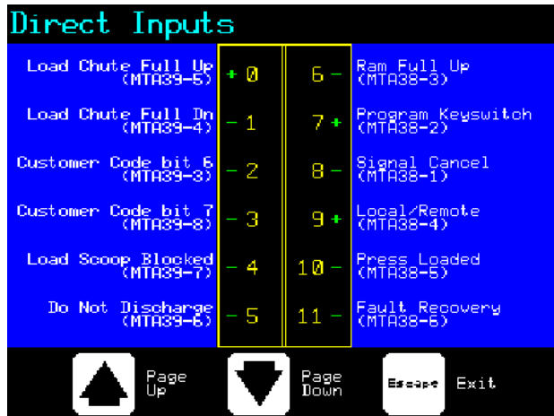
Afbeelding 27: Scherm invoer voor microprocessorkaart
