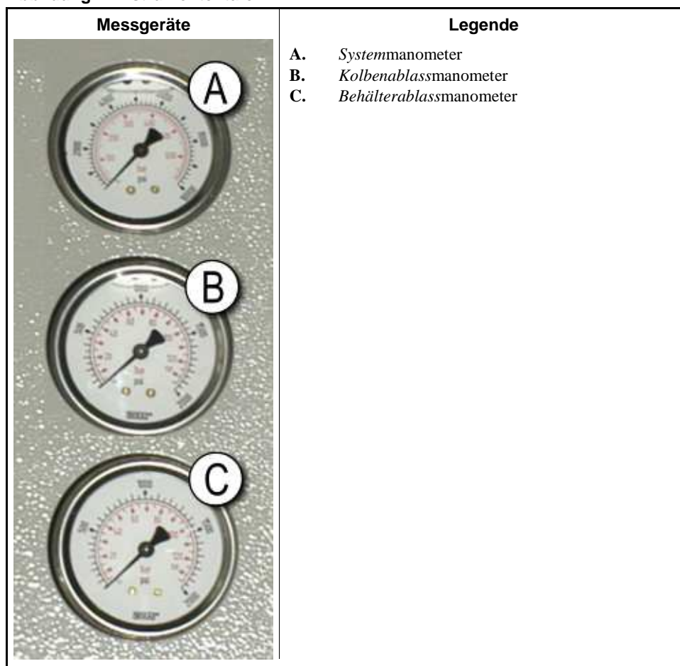
Abbildung 7: Instrumententafel
