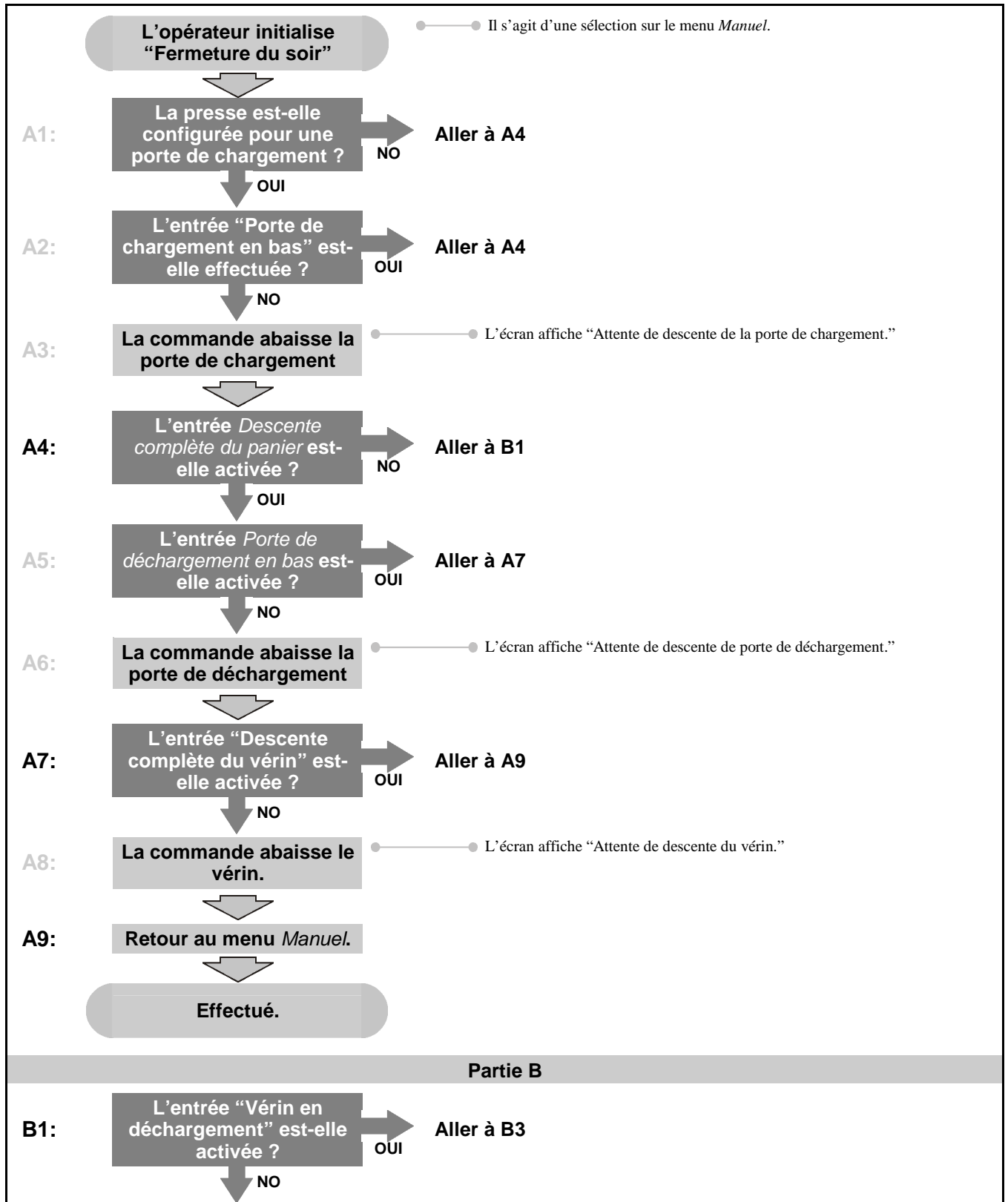
Graphiques 1: Graphique descriptif de la fermeture du soir
