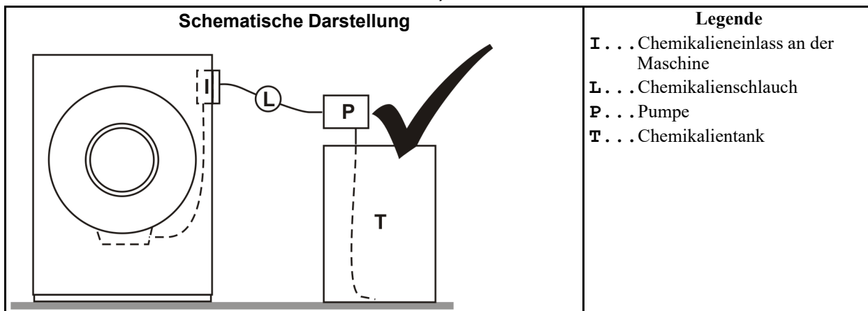
Abbildung 5. Eine Konfiguration, die bei ausgeschalteter Pumpe (d. h. wenn der Chemikalienschlauch und der Tank drucklos sind) einen Durchfluss in der Maschine verhindert
