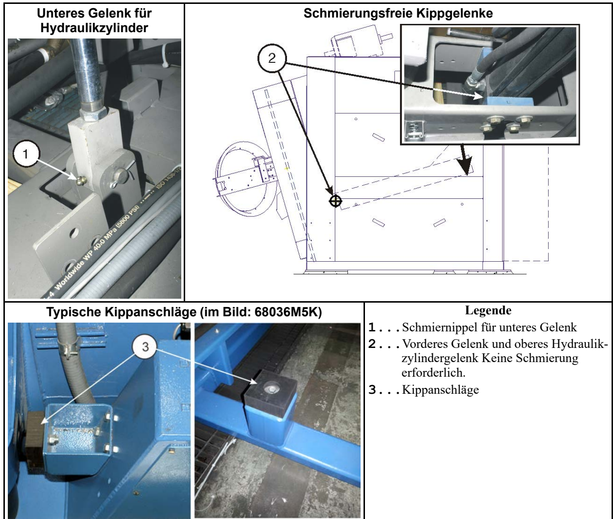
Abbildung 22. Sonstige Punkte der routinemäßigen Wartung auf beiden Seiten der Modelle M_K – Waschschleudermaschine mit hydraulischer Kippvorrichtung
