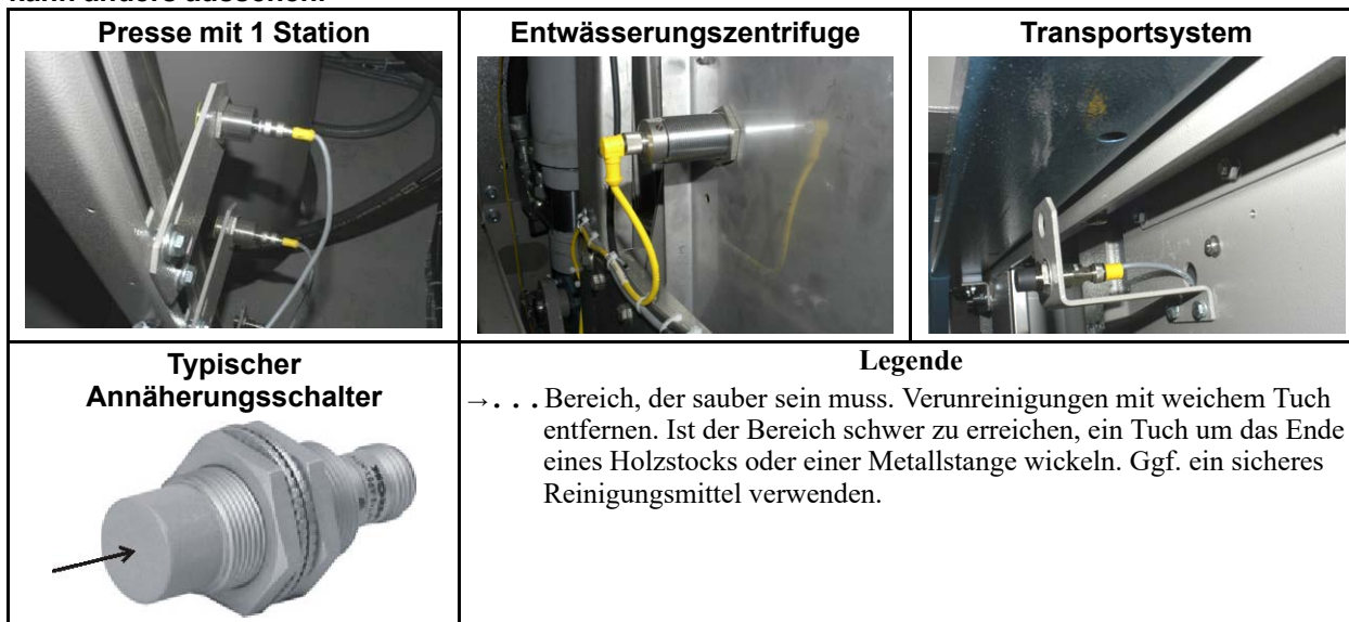
Abbildung 19. Nachstehend sind einige Annäherungsschalter als Beispiel aufgeführt. Ihre Anlage kann anders aussehen.
