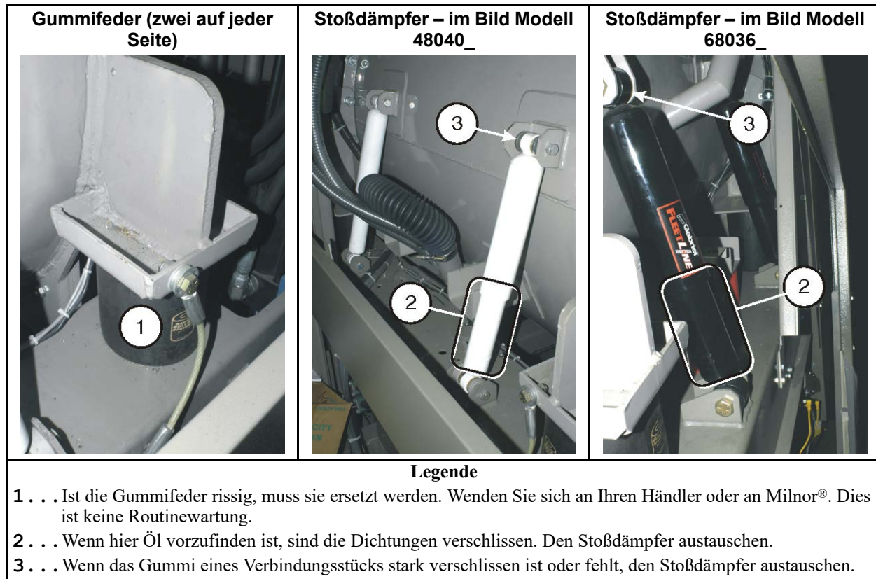
Abbildung 24. Beidseitige Komponenten der Aufhängung einer mit Gummifedern aufgehängten Waschschleudermaschine (siehe Abschnitt 3.3.4 : Informationen zu den Stoßdämpfern, Seite 47 )
