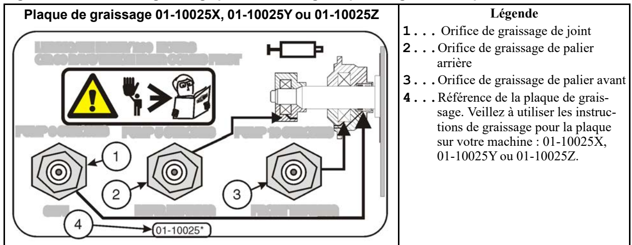
Figure 20. Orifices de graissage pour assemblage de palier à graisse uniquement
