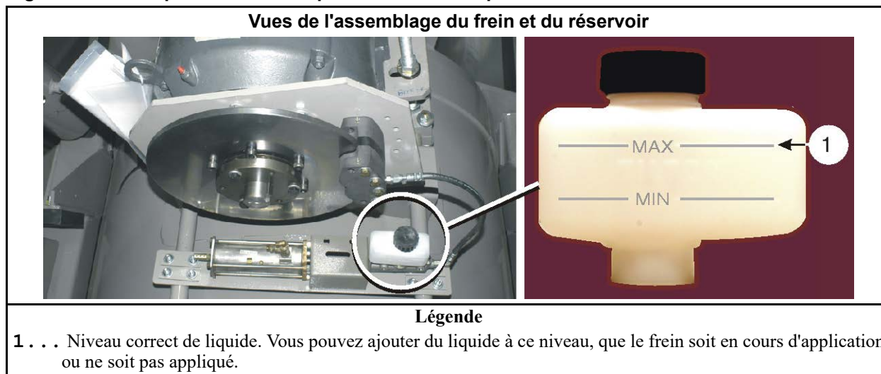
Figure 23. Exemple de frein à disque. Votre machine peut être différente.
