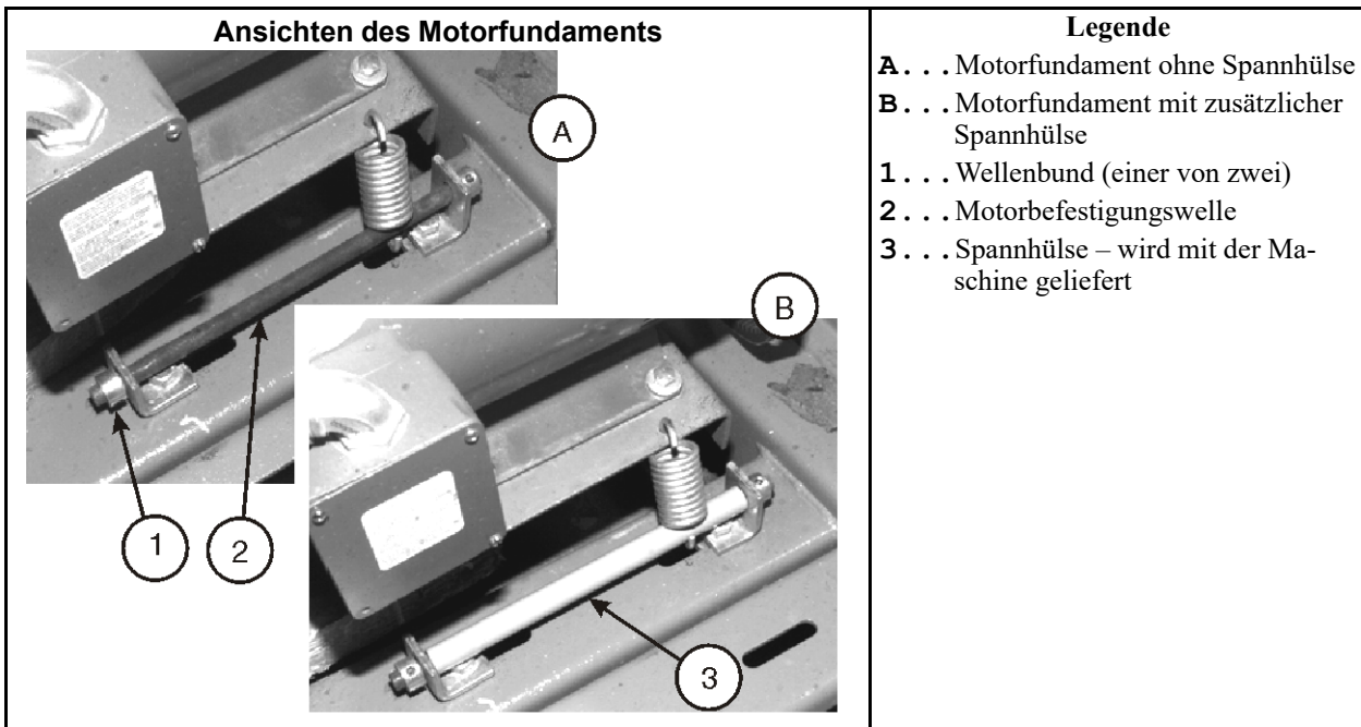
Abbildung 7. Einstellen der Riemenspannung bei Maschinen mit Federvorspannung
